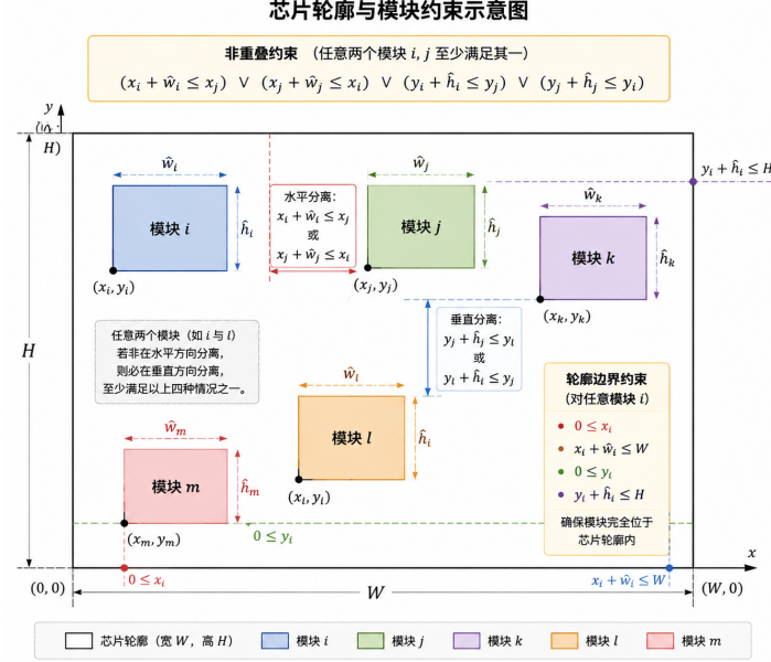
图 5 问题一约束条件示意图
