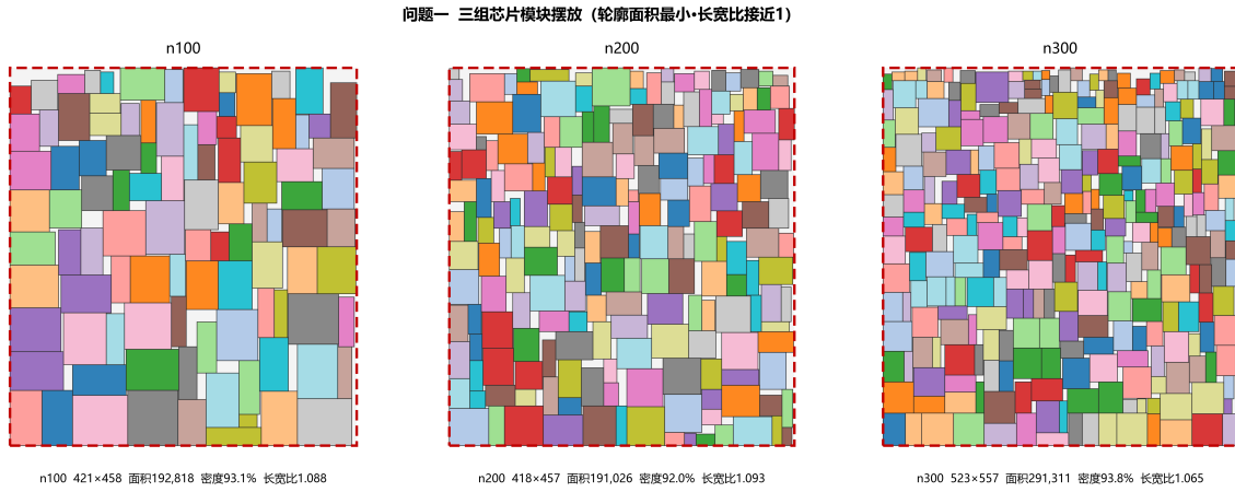
图 7 问题一三组芯片的模块摆放可视化
